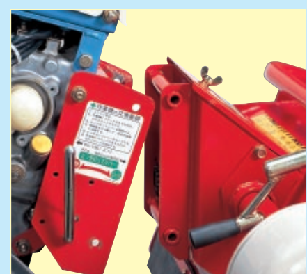
① ティラー側のヒッチを作業機側のヒッチにひっかけます。
